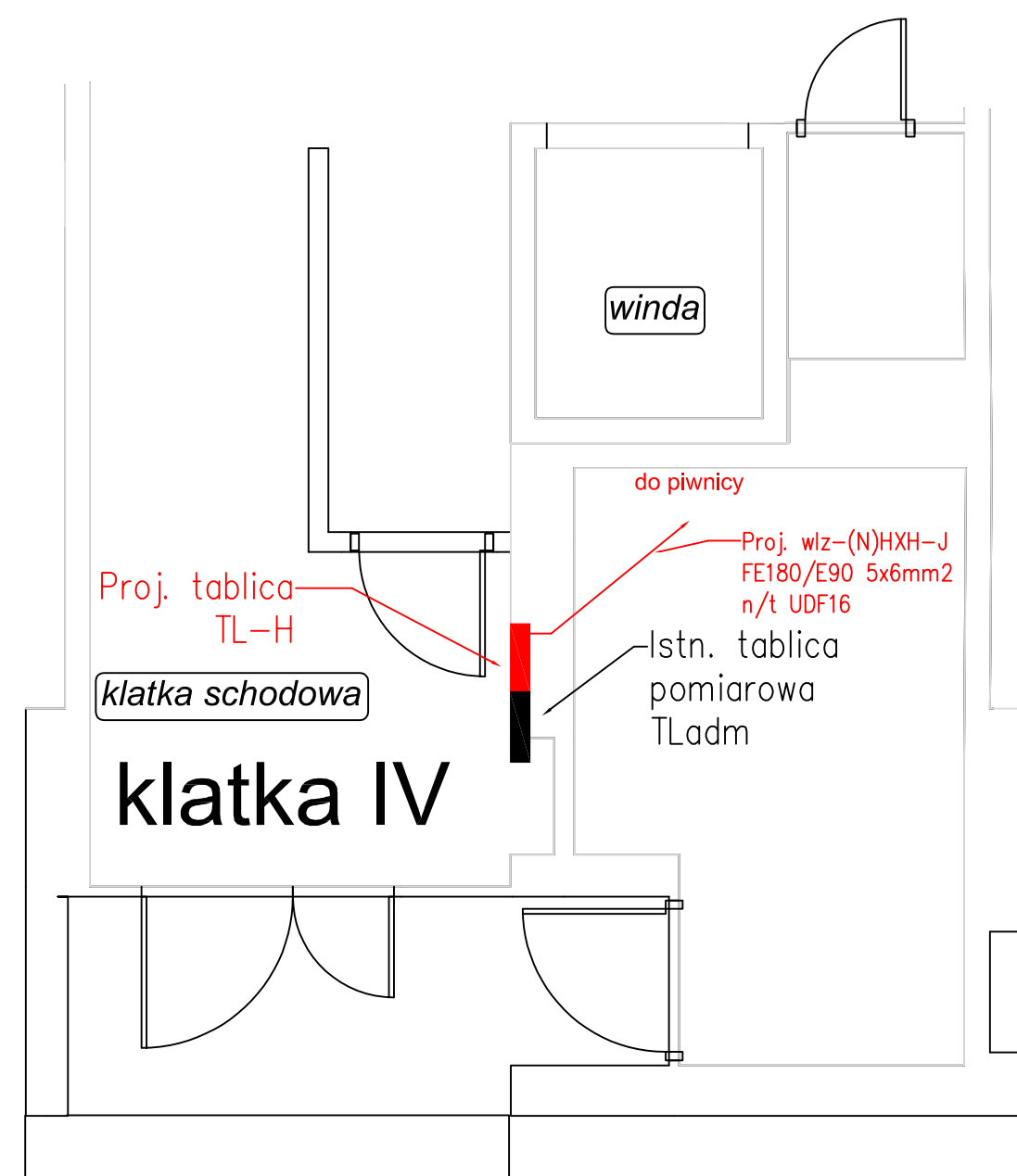
rzut parteru
